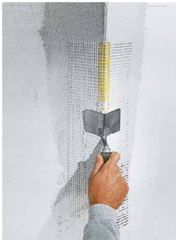
Fig. 16 : Renfort d'angle
