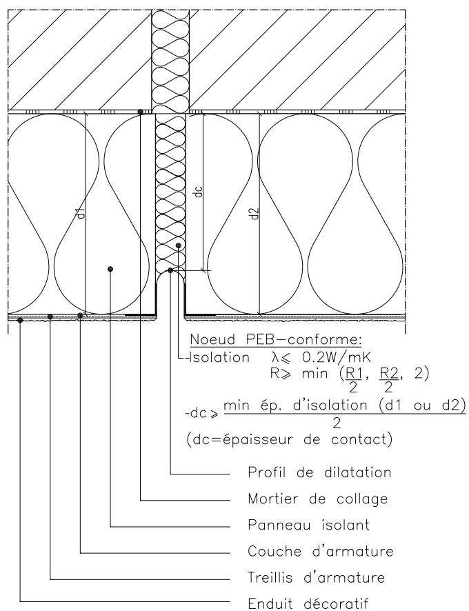
Fig. 18: Joint de dilatation sur la surface
