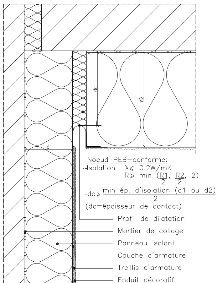
Fig. 17: Joint de dilatation dans un angle
